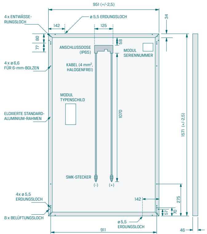
Alle Abmessungen in mm; Modulgewicht 17,4 kg
